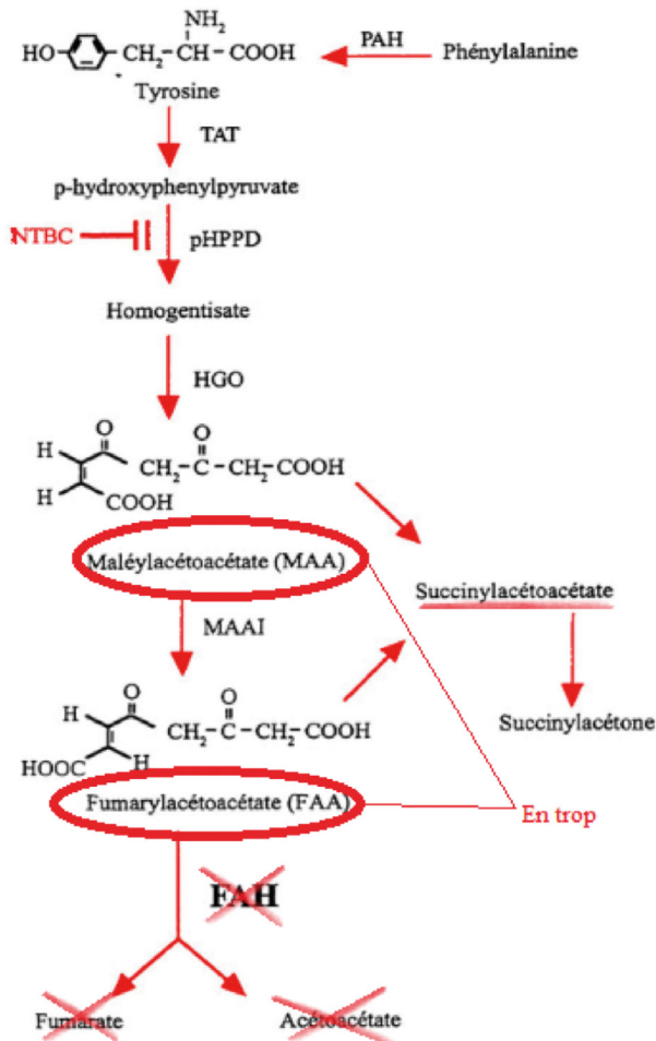
Figure 1. Chaîne catabolique de la tyrosine pour un individu atteint de la tyrosinémie de type I
